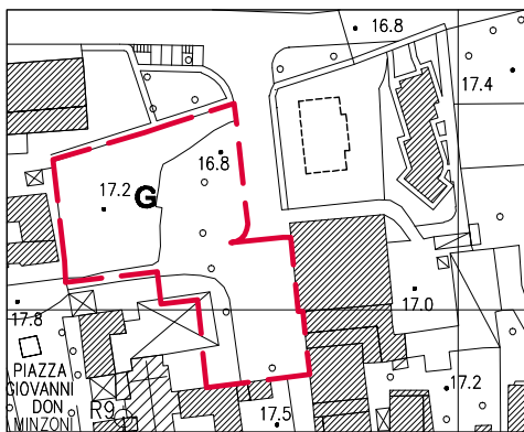
Stato di fatto - Comparto G Scala 1/2000 Superficie del Comparto: 2318 mq.
